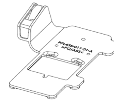
Halteplatte
